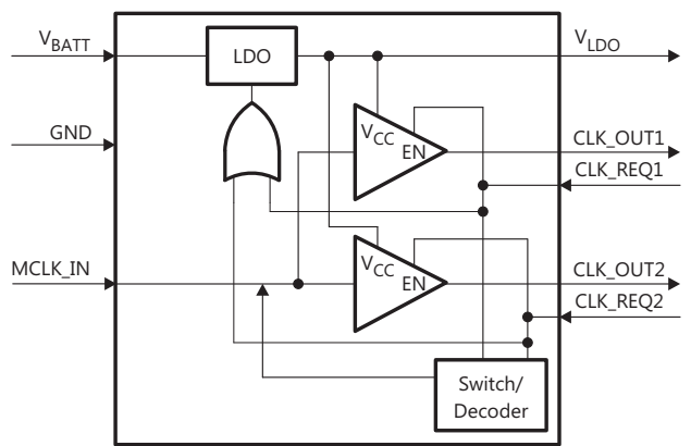
简化框图
